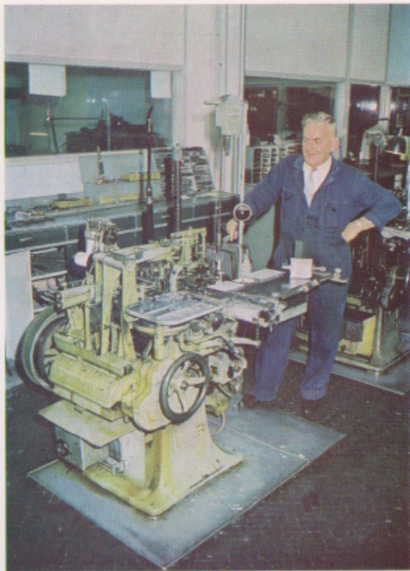
Het gieten van letters
